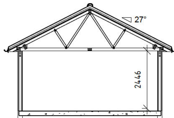
SEKTION A-A
